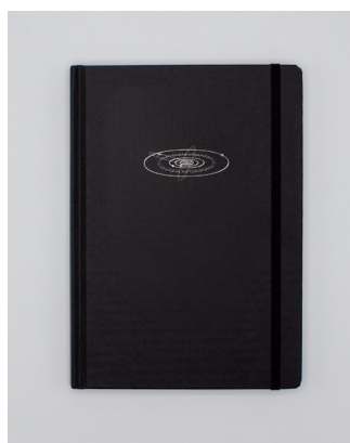
Sol
