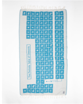
Periodic Table
